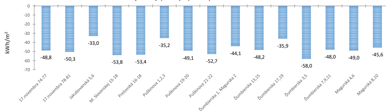
Porovnanie skutočnej mernej spotreby tepla na vykurovanie s normatívom
